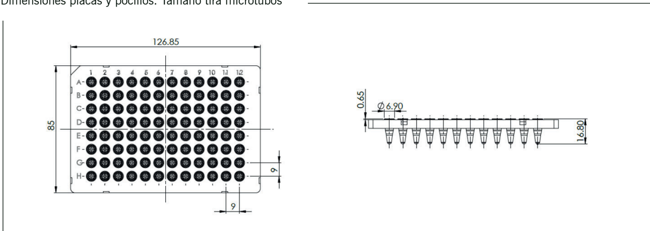
Dimensiones placas y pocillos. Tamaño tira microtubos
